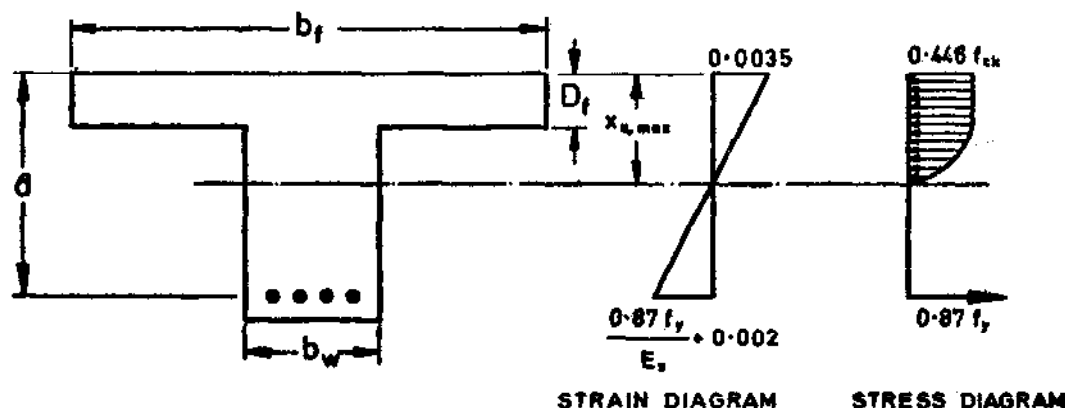
FIG. 6 T-SECTION
